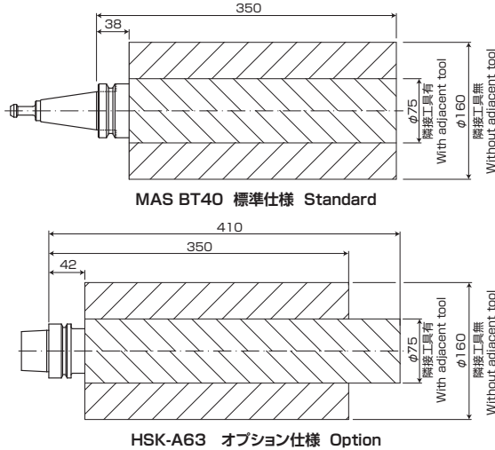
ATC最大工具寸法図 ATC maximum tool dimension
